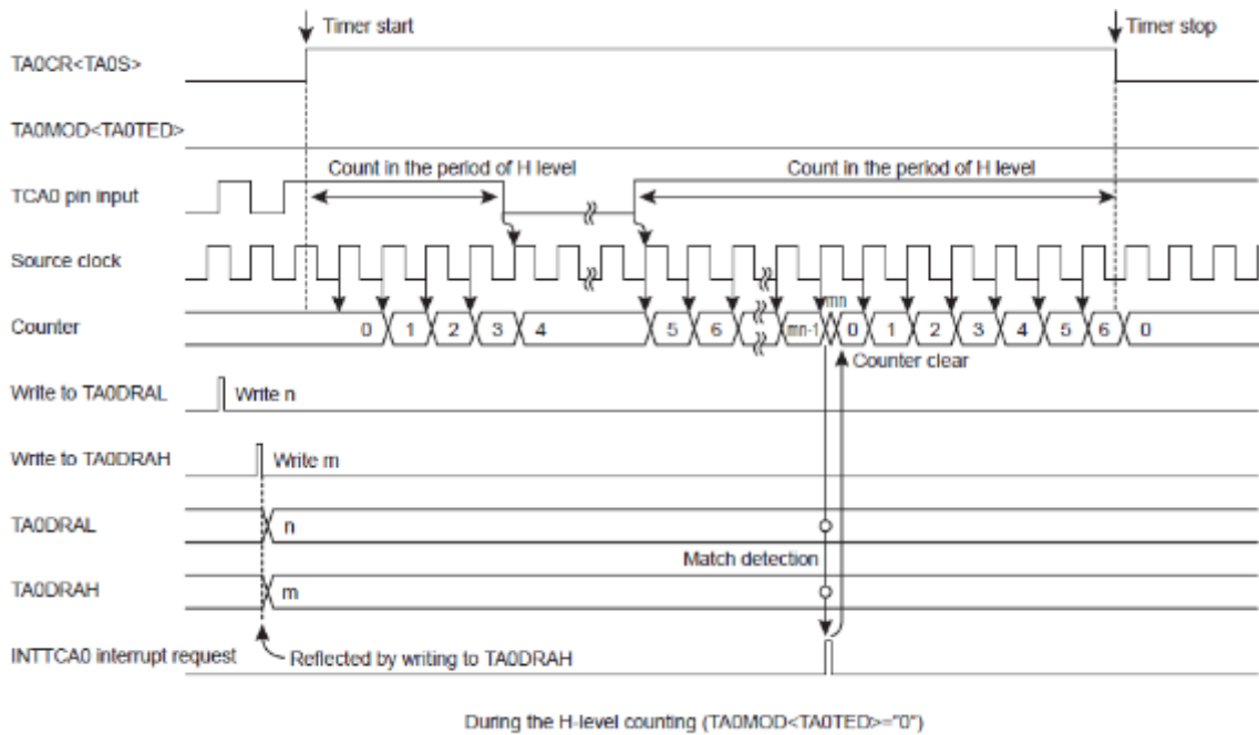
图 10.31 窗模式时序图
