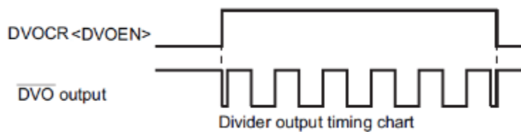
图 10.6 分频器输出时序
