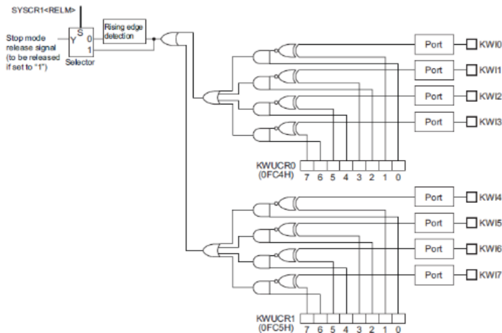
图 4.13 唤醒线路
