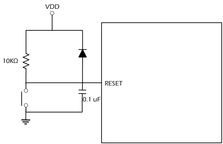
图 2.4 使用 MQ6801 时建议之外部参考线路 (复位引脚)
